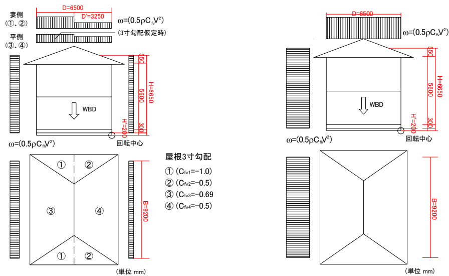
図 1 想定した風圧力分布
