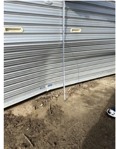
図 6.2.12 変形したシャッター
