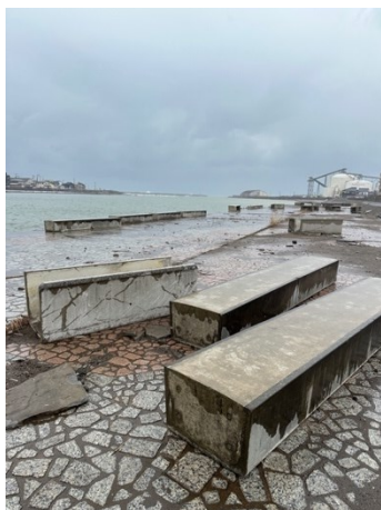
図 4.1.1 コンクリート製のブロックの移動
