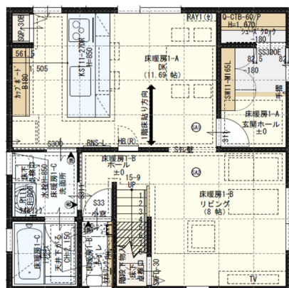
1 階平面図
